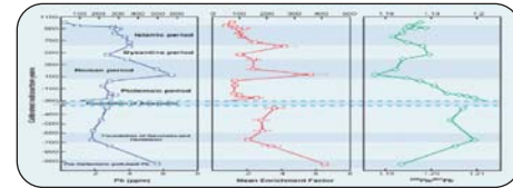
Pollution en plomb à Alexandrie (Egypte) au cours des 3 derniers millénaires. On note sur ces graphiques un pic de plomb vers -900 av. J.-C. soit bien avant la fondation de la ville par Alexandre. L'utilisation de la géochimie du plomb suggère un peuplement préhellénistique du site.
