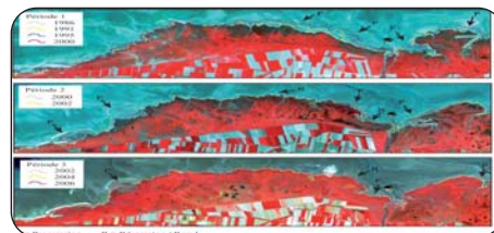
Spatialisation de la limite shore/slikke et évolution entre 1986 et 2006 en trois périodes.
